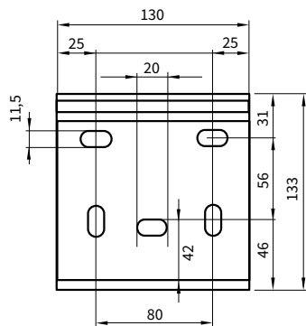
vooraanzicht muursteun
