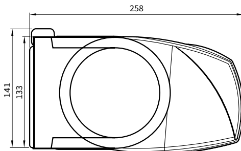
zij aanzicht scherm
