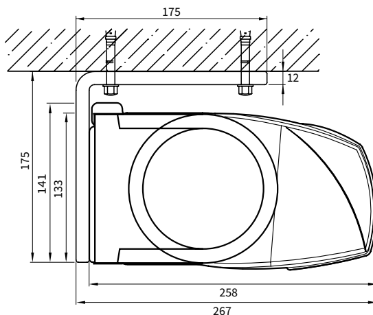
zij aanzicht scherm
