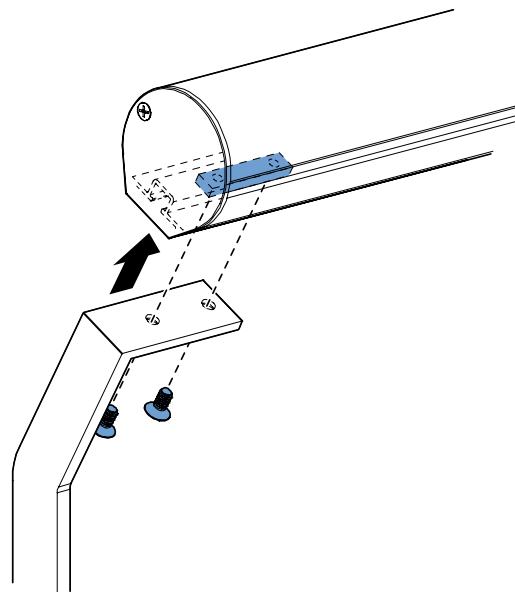
fig. 2.8 Uitvalarm vastschroeven
