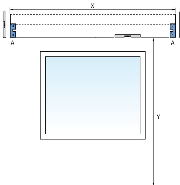
fig. 1.2 Plaatsing muursteunen
