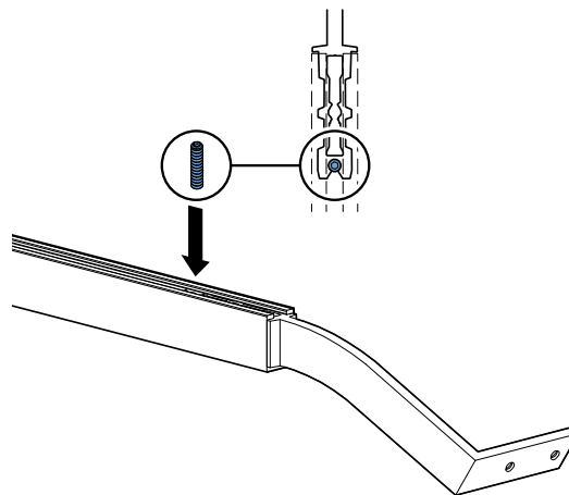
fig. 2.6 Kopstukken vastzetten
