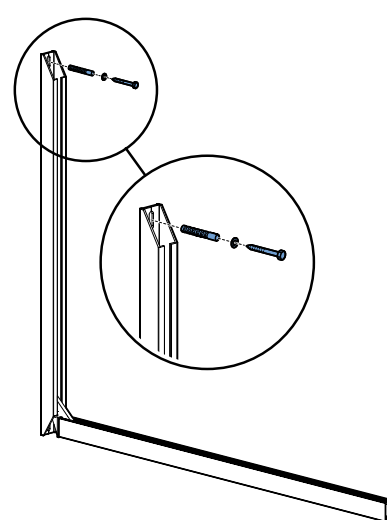
fig. 2.4 Bevestigen uitvalarm boven
