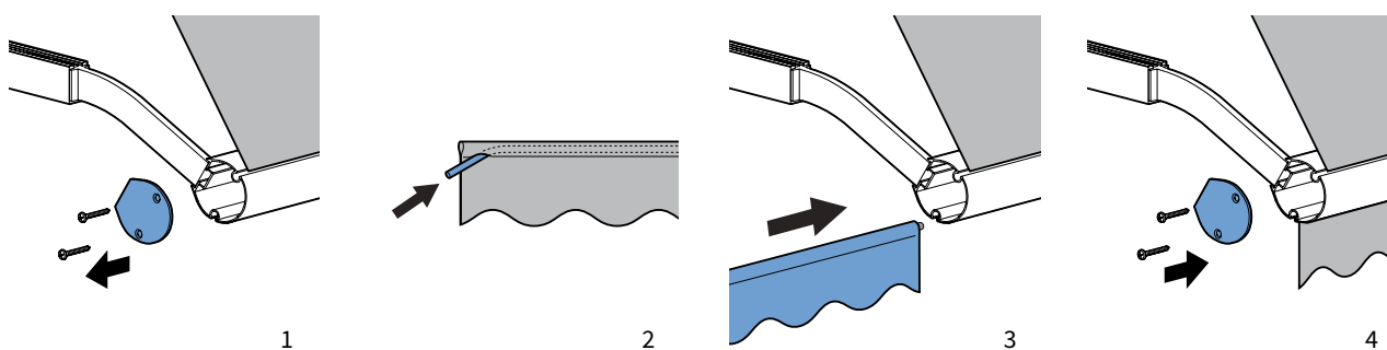
fig. 8.1 Plaatsen volant
