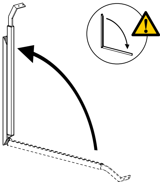
fig. 2.7 Terugklappen uitvalarm
