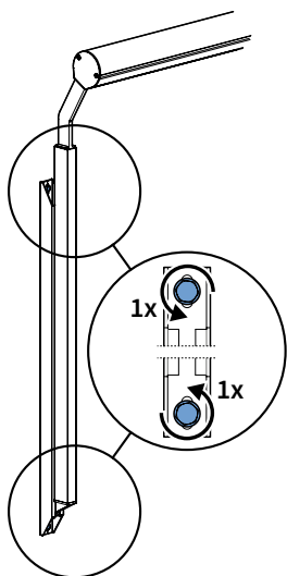
fig. 6.2 Losdraaien bevestigingsbouten
