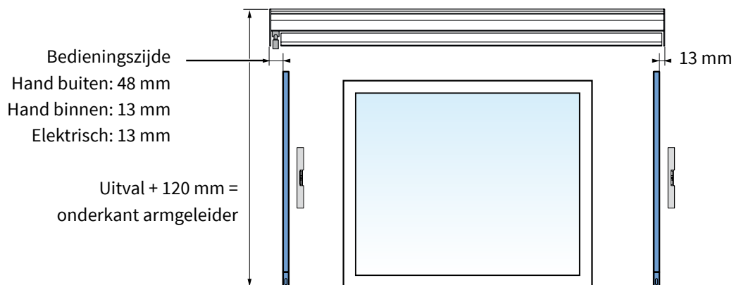
fig. 2.1 Uitmeten uitvalarmen
