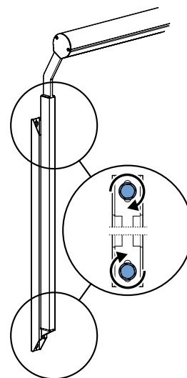
fig. 6.4 Vastdraaien bevestigingsbouten
