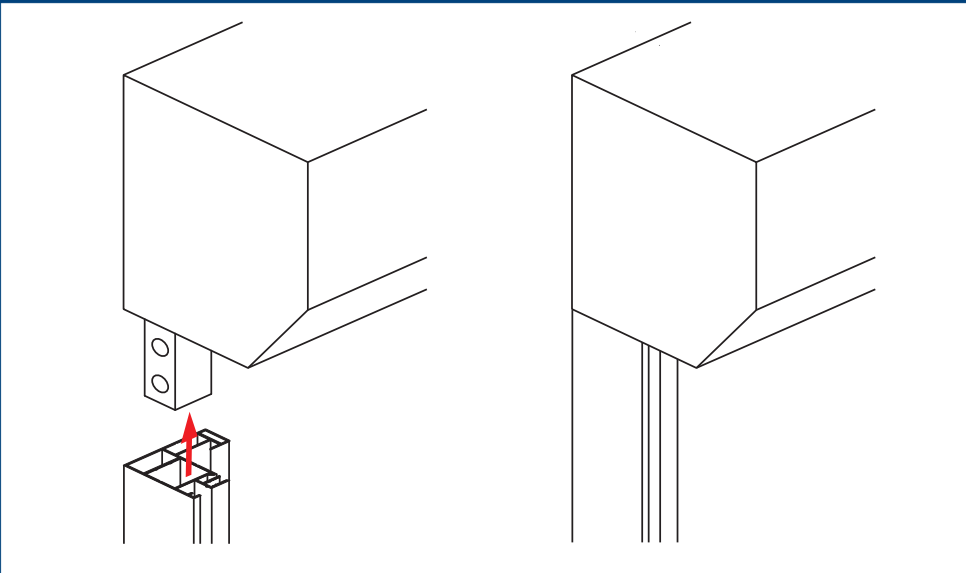
5.8 Schuif de geleiderails op de zijkap pin.
