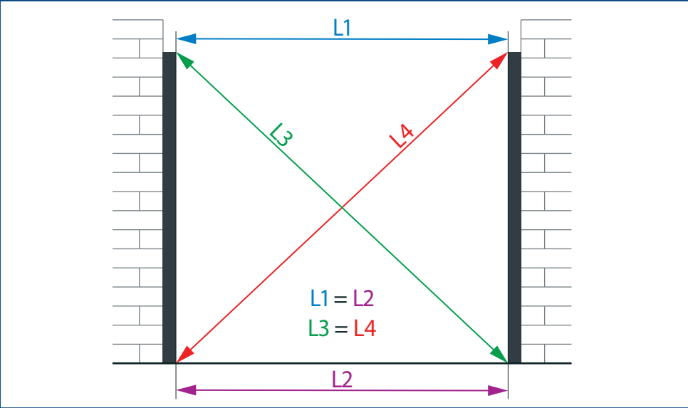
5.11 Controleer de breedte en de diagonalen.
