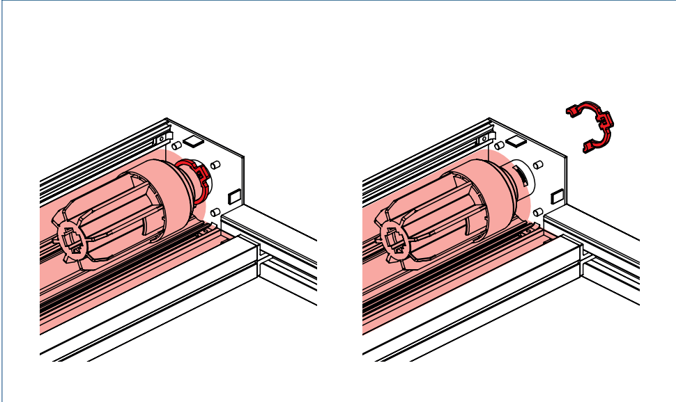
5.15 Monteer de pen op de asprop.
