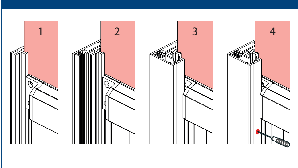
8.13 (1) Steek het doek in de inlays. (2) Monteer de inlays op de geleiding. (3) Monteer de voorkant van de geleiders. (4) Schroef deze vast.
